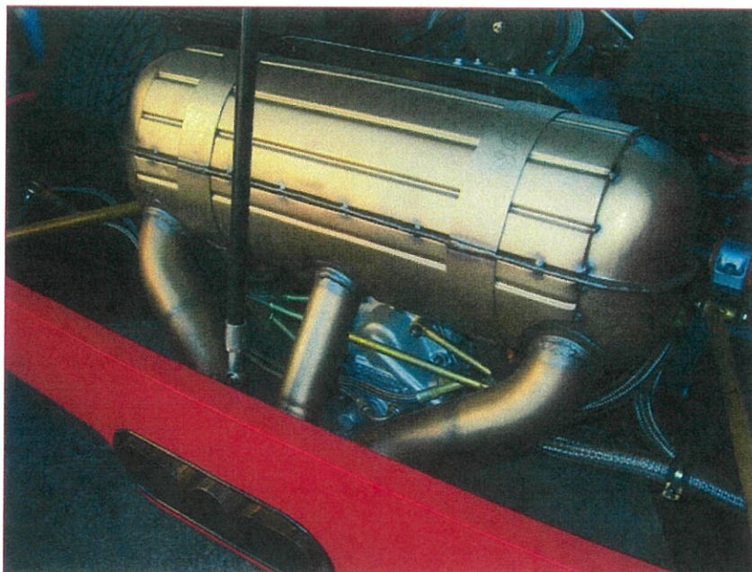
Impianto di scarico Exhaust system
