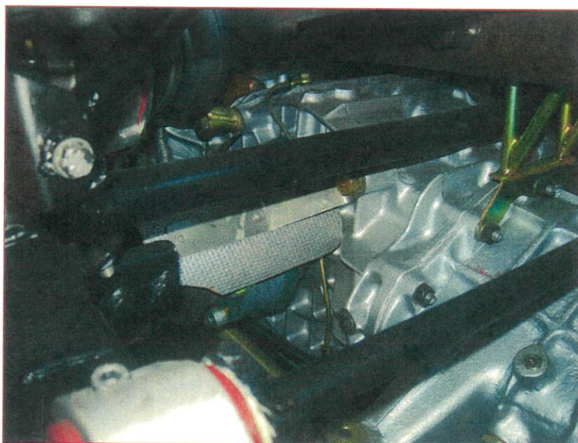
Foto differenziale in vettura (solo nel caso i gruppi siano divisi) Picture of the differential in the car (if the gearbox/differential units are separated)
