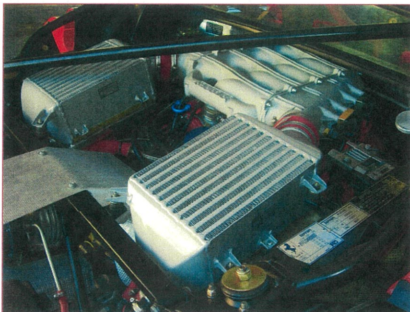
Motore - vista lato destro
