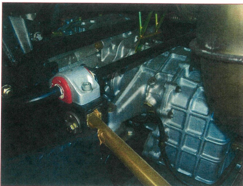
Foto cambio/differenziale in vettura (nel caso i gruppi siano divisi, riportare la fotografia del cambio) Picture of the gearbox/differential unit in the car (if these units are separated please show the picture of the gearbox)
