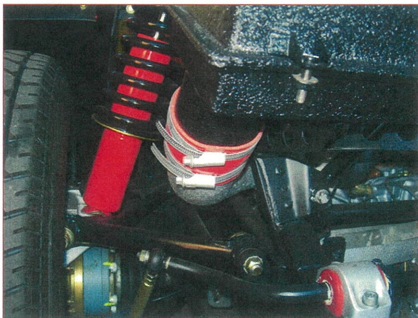
Sospensione posteriore
