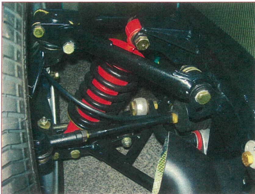
Sospensione anteriore
