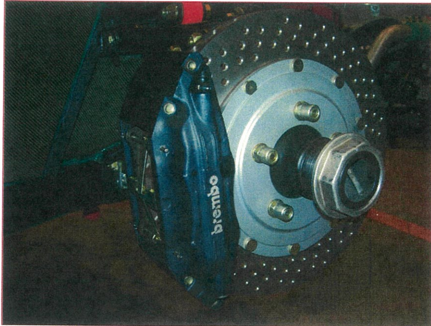
Assieme freno ruota anteriore
